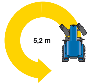
Oś 4WD
